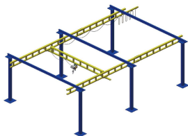
欧式刚性起重机FEM Light Duty Crane
